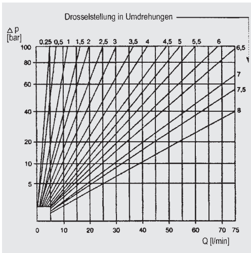
Typ DVG 10
