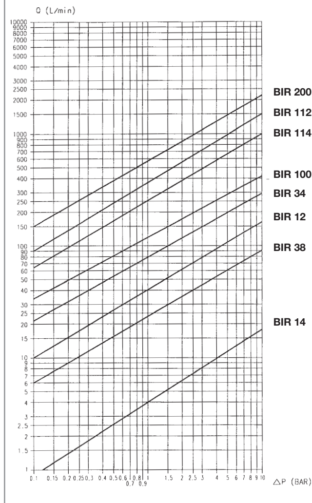
Durchflussdiagramm
