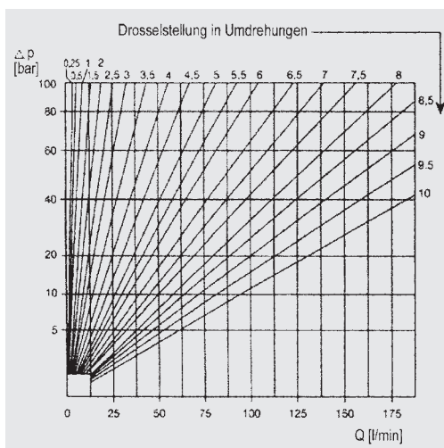
Typ DVG-R 16
