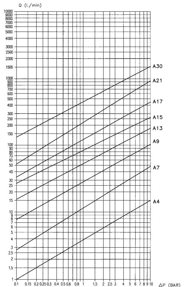
Durchflussdiagramm
