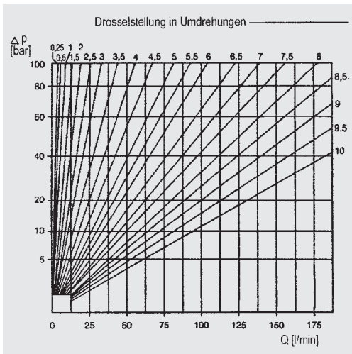
Typ DVG 16
