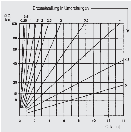
Typ DVG 8
