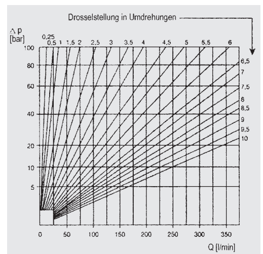
Typ DVG-R 20/25/ 30/40
