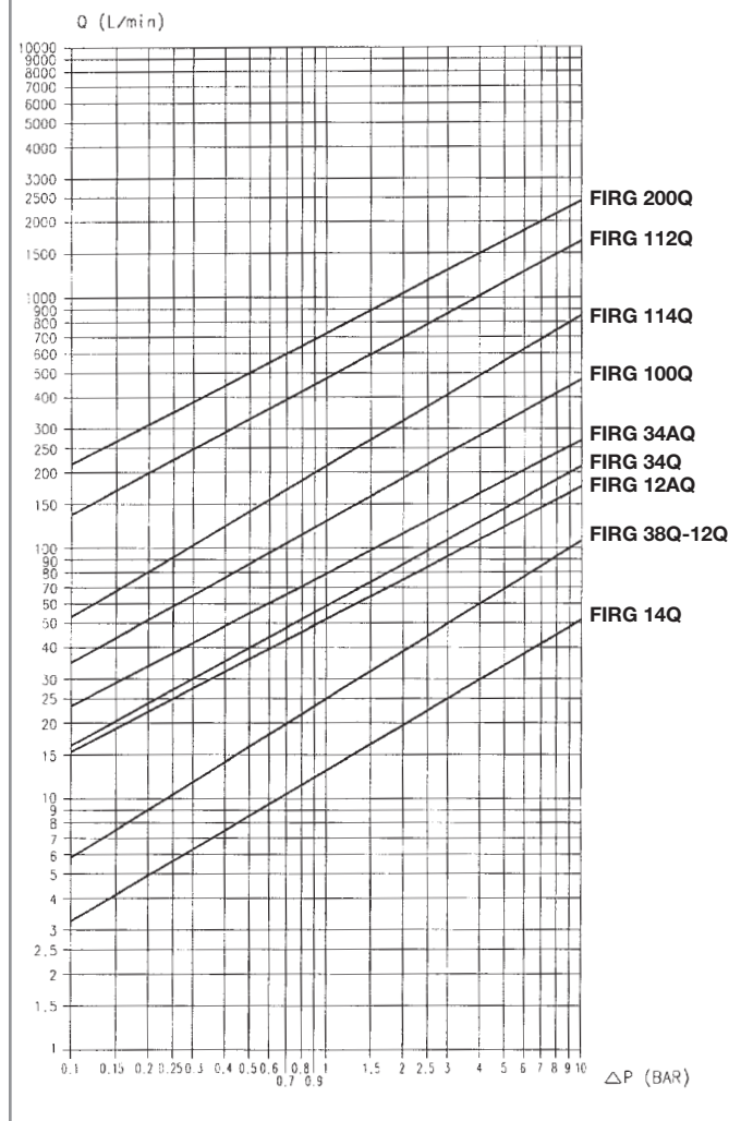
Durchflussdiagramm
