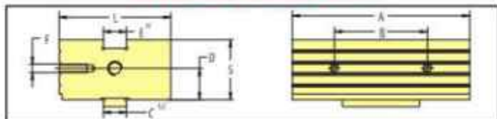
CORPO FISSO 1 GRADINO/FIXED BODY WITH 1 STEP E.G. 99
