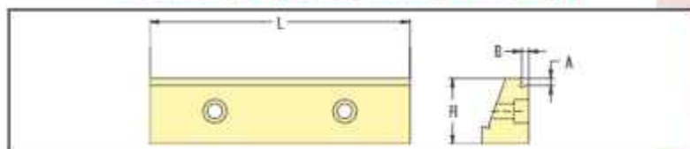
GANASCIA A V/V-JAW SPE. 81
