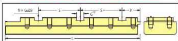
GUIDA CARRO/TROLLEY GUIDE ES-ET03
