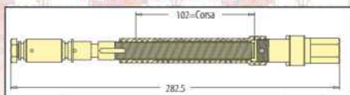
GRUPPO VITE/SCREW UNIT GR 76
