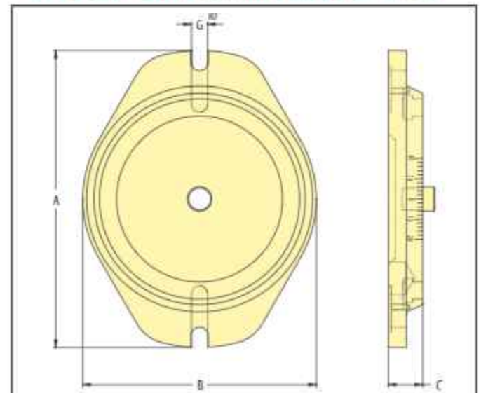
BASE GIREVOLE/ ROTATING BASE AC - PIA 83
