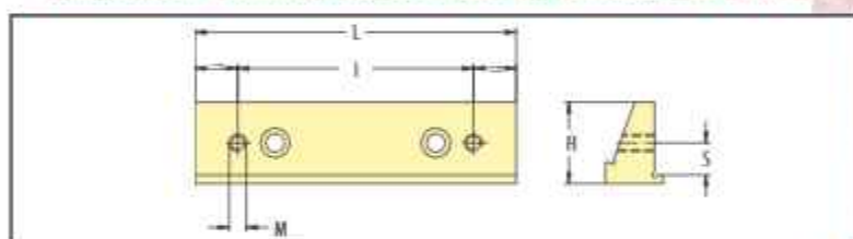
BLOCCHETTO TENERO/SOFT BLOCK SPE. 81
