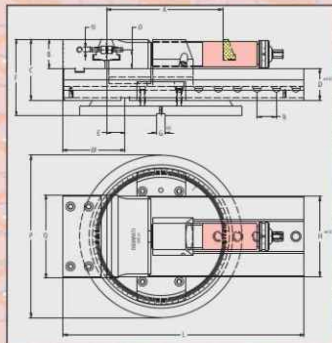
TIPO / TYPE ISPE. - MSPE. 81
