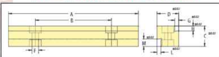
GANASCIA A GRADINO/STEPPED JAW E03
