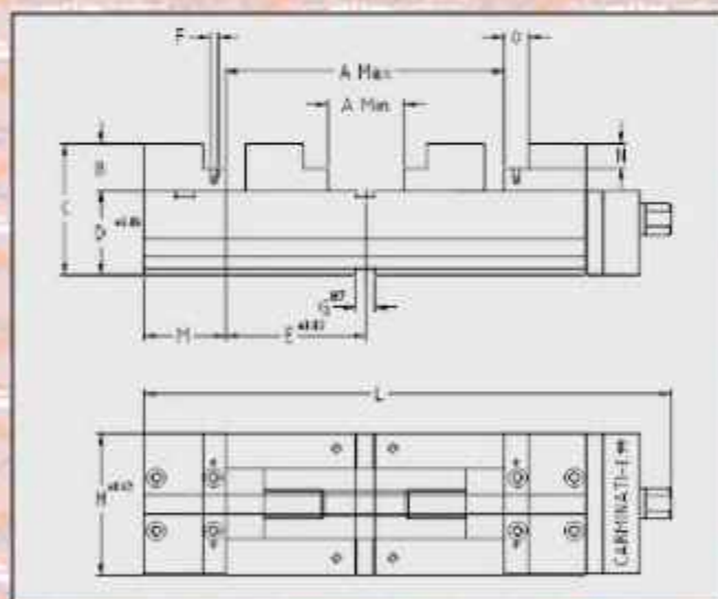
TIPO / TYPE EGA.99
