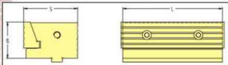
FISSO/FIXED SPE. 81
