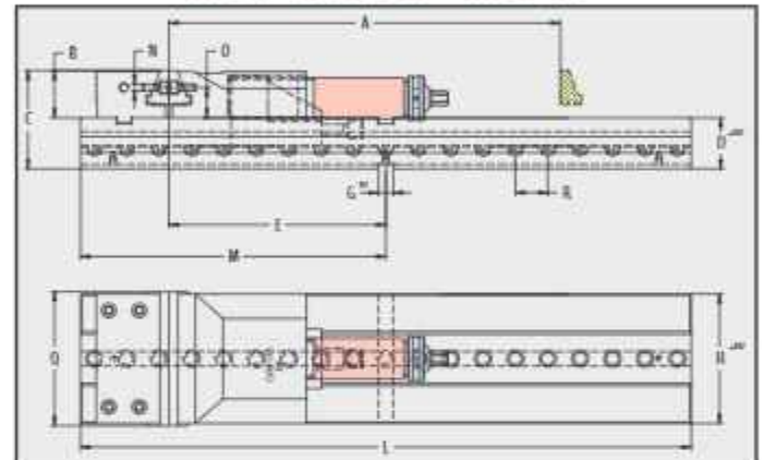
TIPO / TYPE IPSP - MPSP 81
