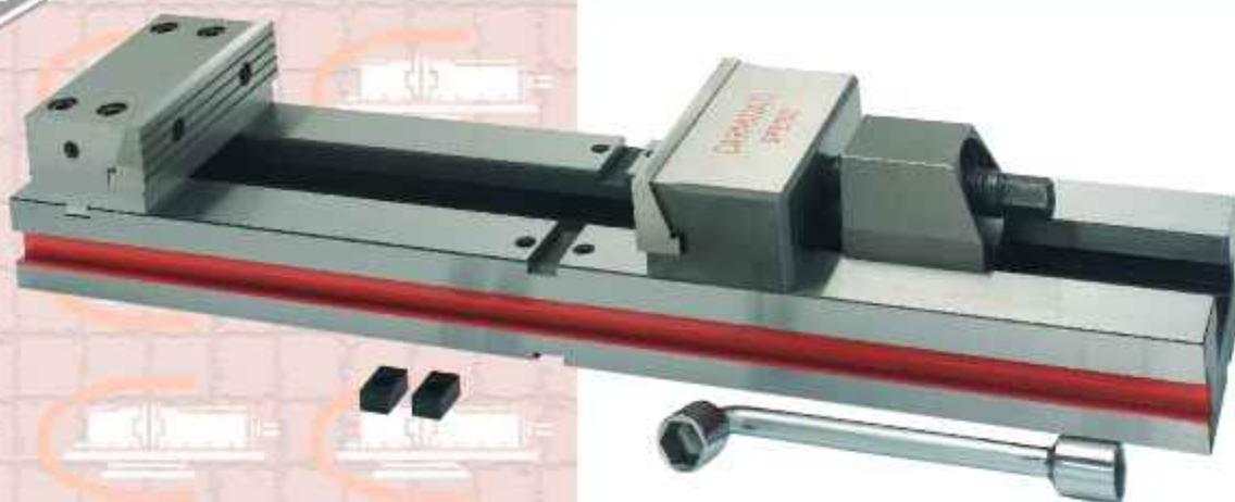
TIPO / TYPE IPSPE. - MPSPE. 81
