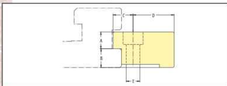
STAFFE PIATTELLO/PLATE BRACKETS SPE. 81
