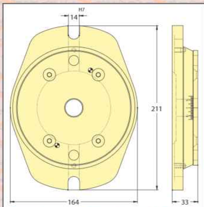
GANASCIA A V/V-JAW GR 76
