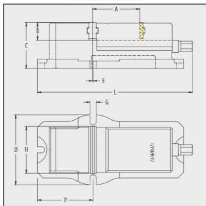
TIPO / TYPE GR 76
