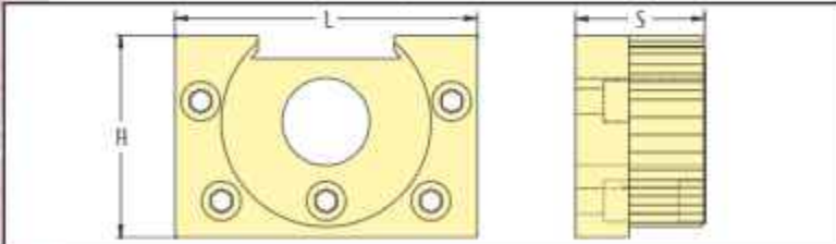
GANASCIA A GRADINO/STEPPED JAW E03
