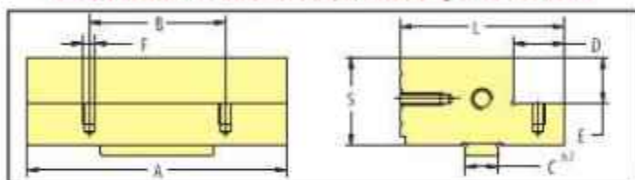
CARRELLO 1 GRADINO/TROLLEY, 1 STEP E03
