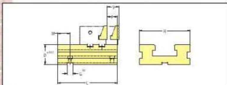
PROLUNGA FISSA/FIXED EXTENSION SPE. 81
