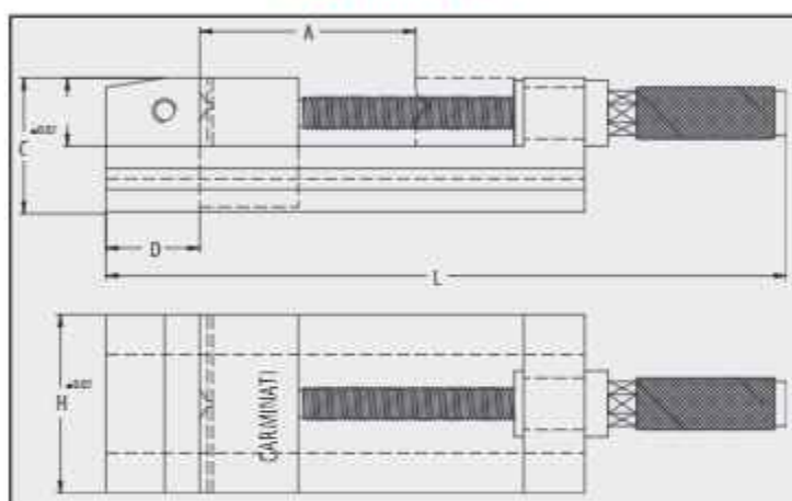
TIPO / TYPE PR. 79
