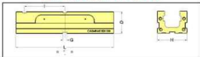
CORPO MORSA/VICE BODY E03
