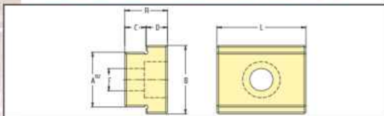
GUIDA RIFERIMENTO/REFERENCE GUIDE SPE. 81
