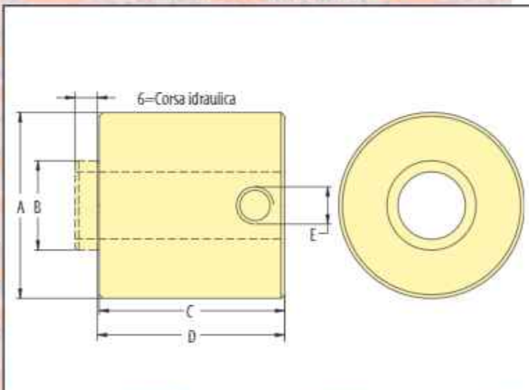
CILINDRO/CYLINDER PIA 83
