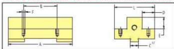
CORPO FISSO 2 GRADINI/FIXED BODY WITH 2 STEPS E03
