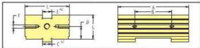
CARRELLO/TROLLEY E. 99
