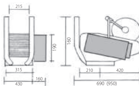
El-drevet garnspil. Idéel til mindre både / Electrically driven nethauler. Ideal for smaller boats.
