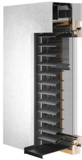
Bautiefe 170*
