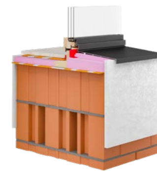
Ziegelmauerwerk verputzt
