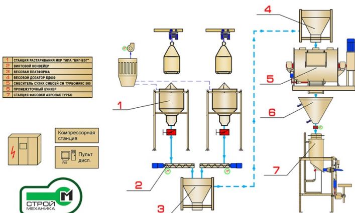
МИНИ-ЗАВОД ДЛЯ ПРОИЗВОДСТВА СУХИХ СТРОИТЕЛЬНЫХ СМЕСЕЙ ТУРБОМИКС 500 (ДЛЯ НАЧИНАЮЩИХ ПРОИЗВОДИТЕЛЕЙ И ДЛЯ СОБСТВЕННЫХ НУЖД ПРЕДПРИЯТИЙ)
